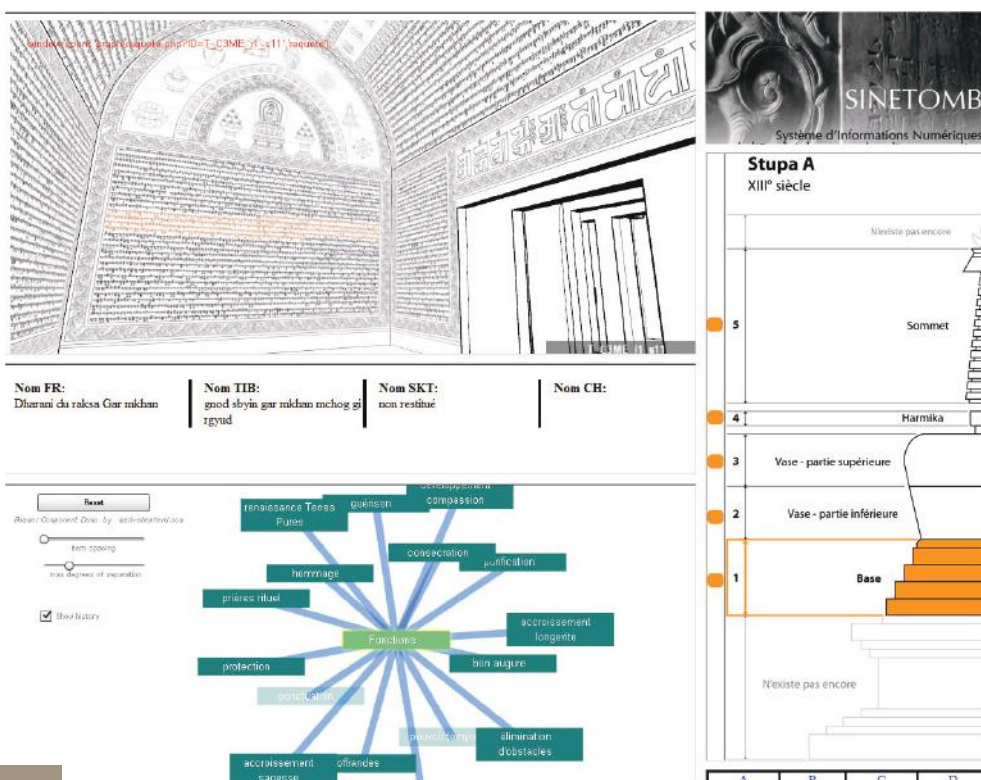
Figure 3 – Interface du système d'informations 3D : en haut, une scène 3D interactive permet la navigation au sein de la représentation de la tombe ainsi que la sélection d'inscriptions ou de sculptures ; au milieu, une barre d'informations contient toutes les traductions des inscriptions sélectionnées ainsi que des sources documentaires annexes ; en bas, le graphe interactif permet l'exploration des entités conceptuelles relatives au rituel funéraire ; à droite, la représentation d'un stupa montre, à chaque sélection d'inscription, le niveau correspondant au sein de sa structure. © MAP / CRCAO
